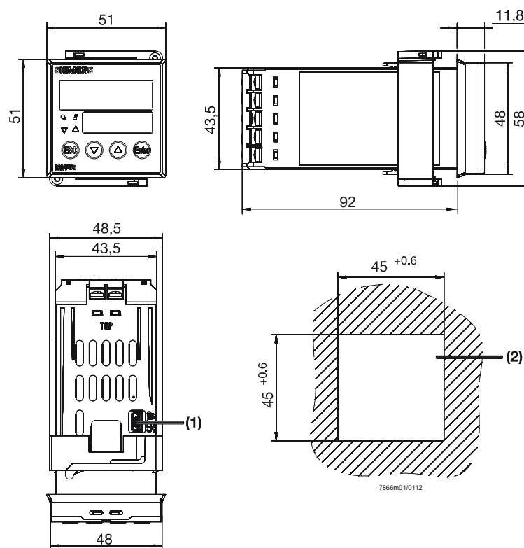
Figura 2: Dimensiones del RWF50
