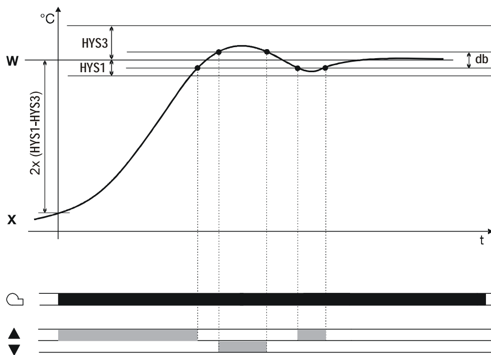
Figura 14: Secuencia de control del arranque en frío de una instalación
