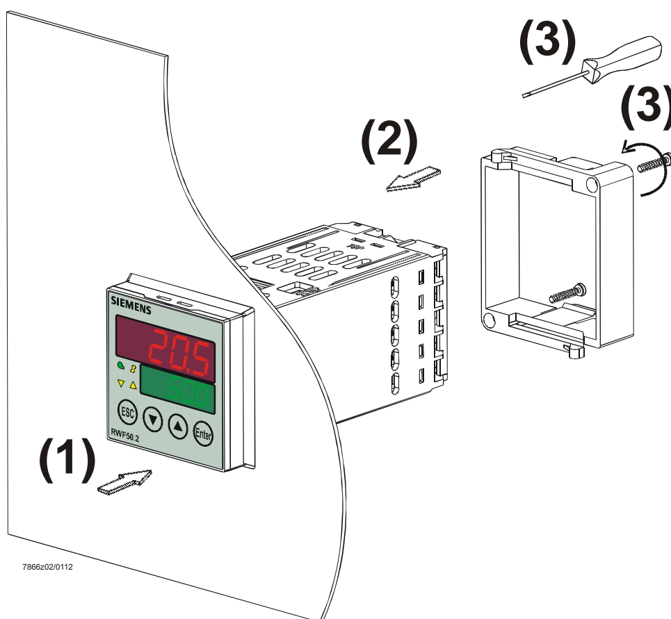
Figura 3: Montaje en abertura de cuadro de mando
